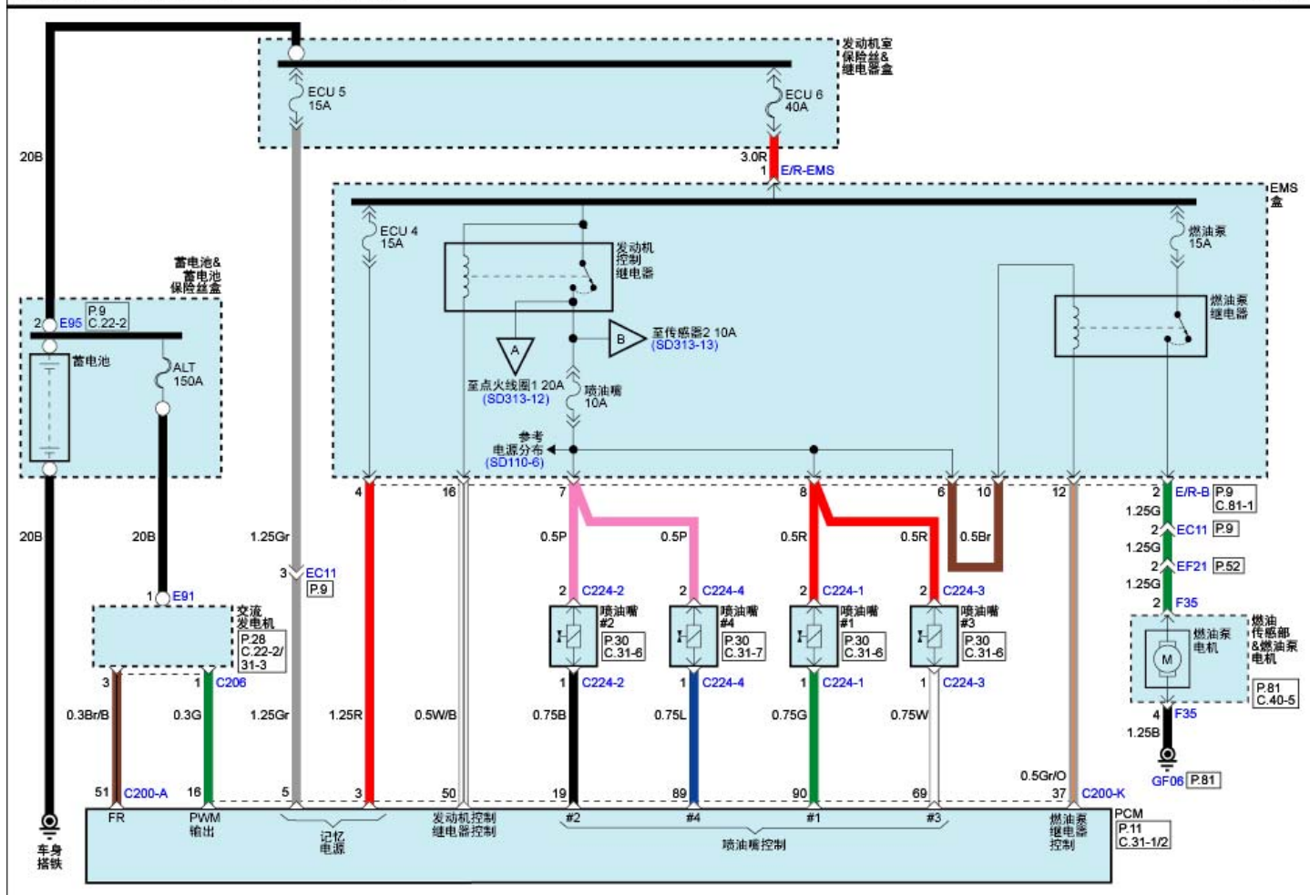
发动机控制系统(G4NB: NU 1.8L MPI)(3)
